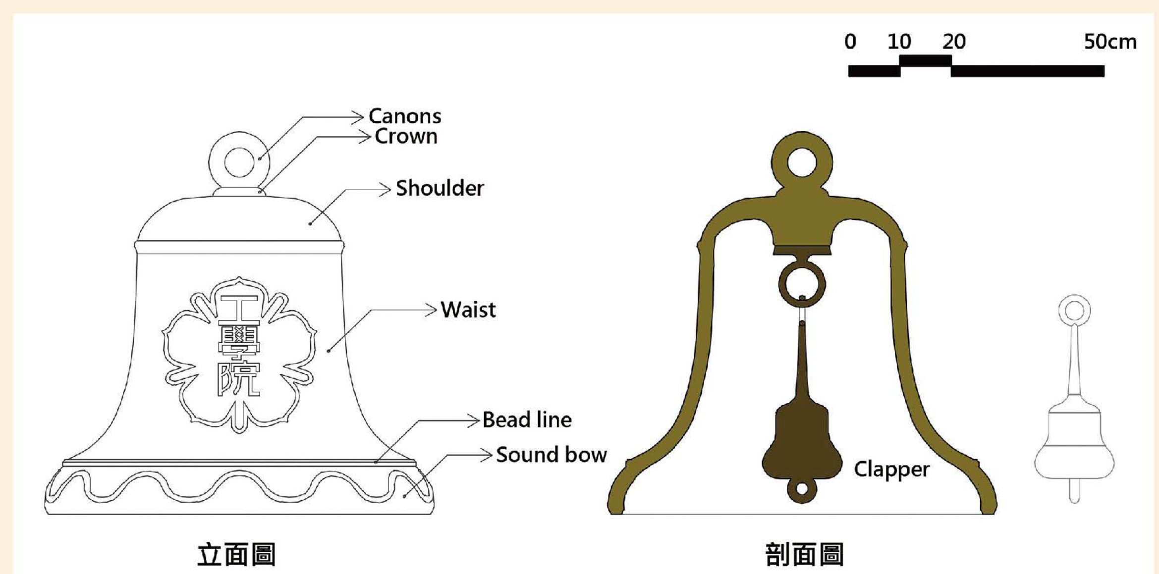
校史文物專輯編纂，繪製之校鐘剖、立面圖
